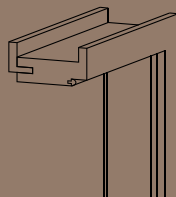
ościeżnica regulowana (zakres regulacji 2cm)
